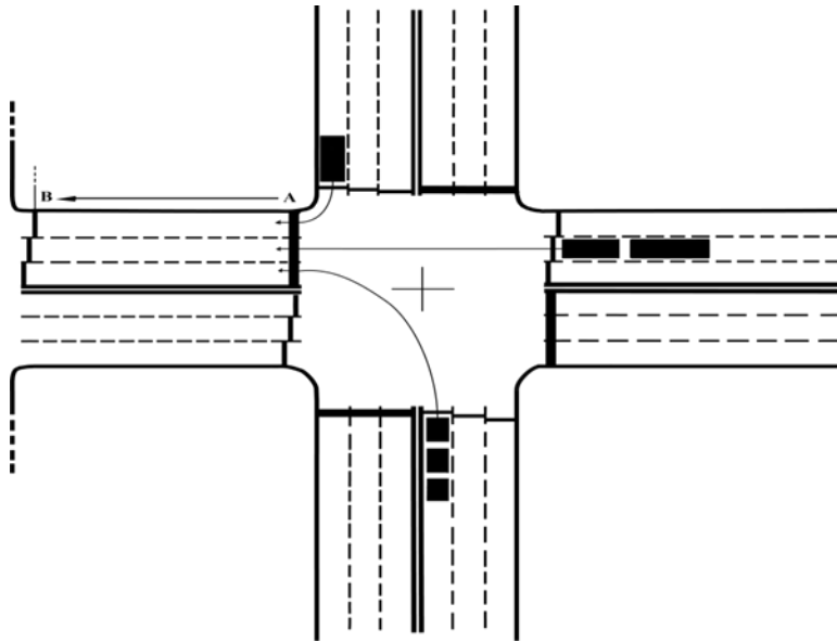
Рис.1. Перехрестя А, з'єднане з сусіднім перехрестям В. Чорними прямокутниками зображені ТЗ, маршрути яких пролягають в напрямку А → В. Показані також вхідні (чорна смужка, позначена літерою А) та вихідні датчики (три рядом розташовані смужки, позначені літерою В). Кожен вхідний та вихідний датчики з'єднані з ВОК (на рисунку зображений лише один такий сигнальний провід, що виходить від одного із датчиків В – це суцільна лінія, що переходить в пунктирну).
